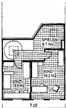
2. OBERGESCHOSS
